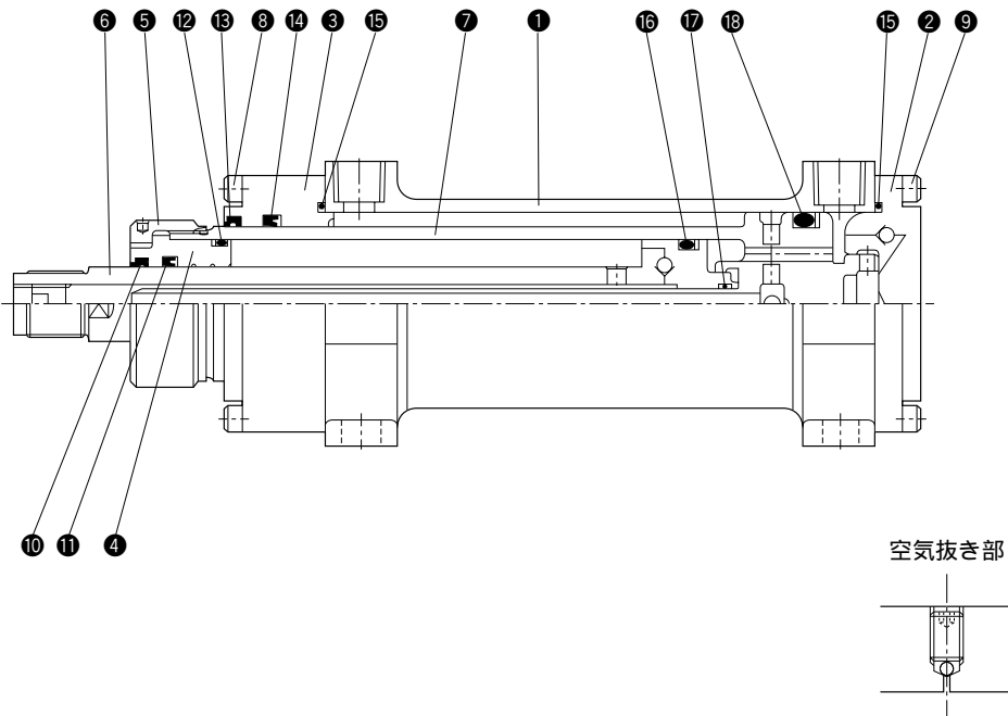
複動形2段テレスコピングシリンダ / 70T-2
