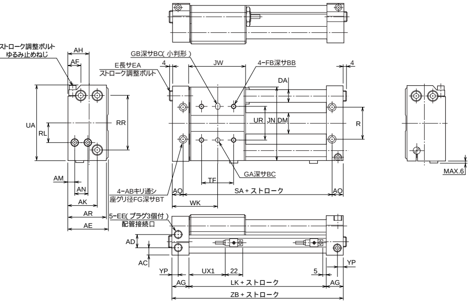
寸法表
