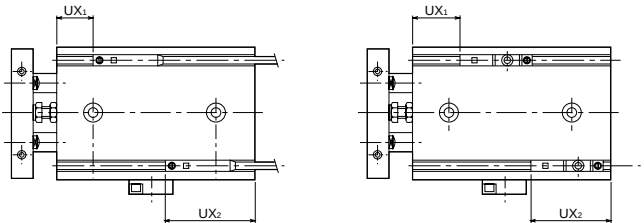
寸法表 / 複動形横ポート
